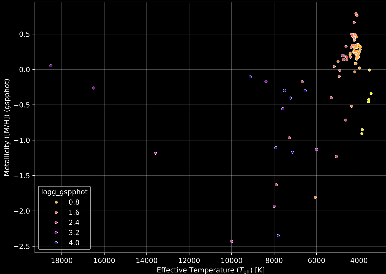
APOGEE DR17 Field: [277-32-O] Stellar Population Parameters (n= 91)
